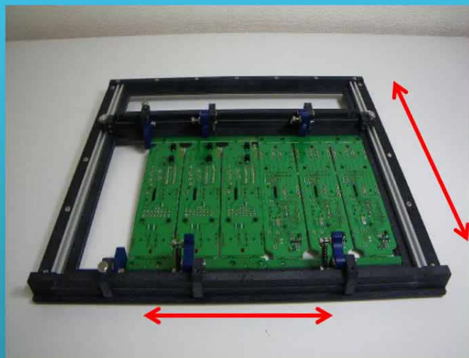
X・Yスライド機構(無段階固定)
